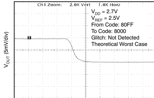
GLITCH ENERGY: 2.7V, 256LSB STEP, FALLING EDGE
